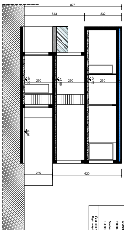
SEZIONE 11
