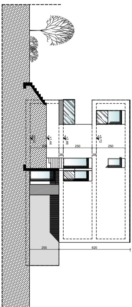
FACCIATA SUD
