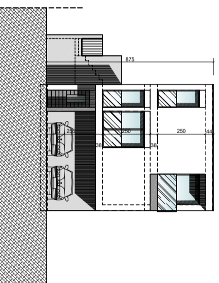
FACCIATA EST
